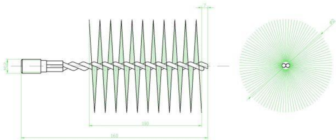
Kominický kartáč kulatý – rozměry
